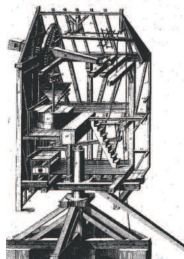
Schemat młyna
